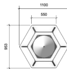
bovenaanzicht
