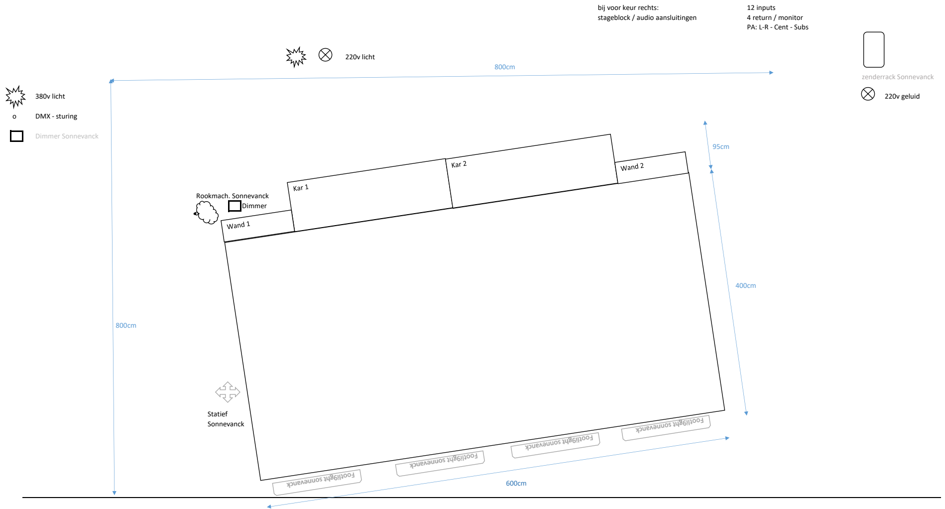
Vloerplan 'Barbaartje' Theater Sonnevanck techniek Jeroen van Terheijden: 0650260943
